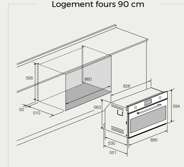
Logement fours 90 cm
