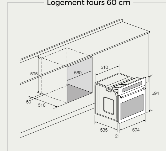
Logement fours 60 cm
